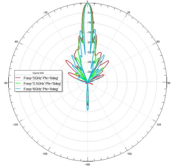
E-plane V-pol
