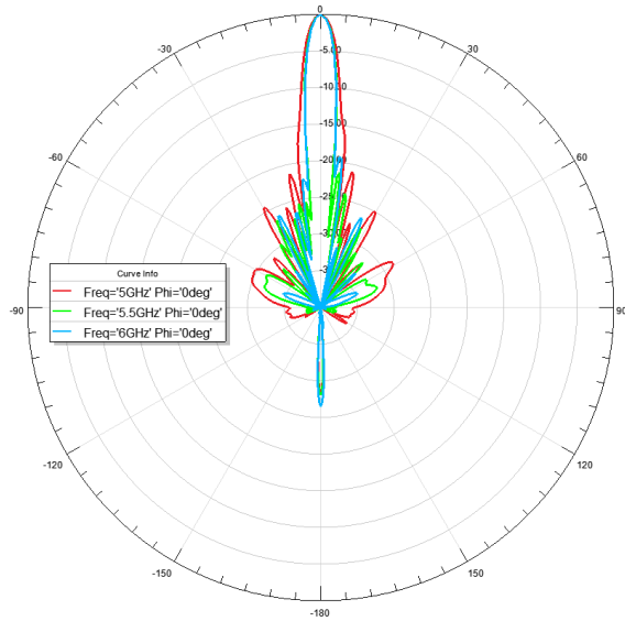
E-plane H-pol
