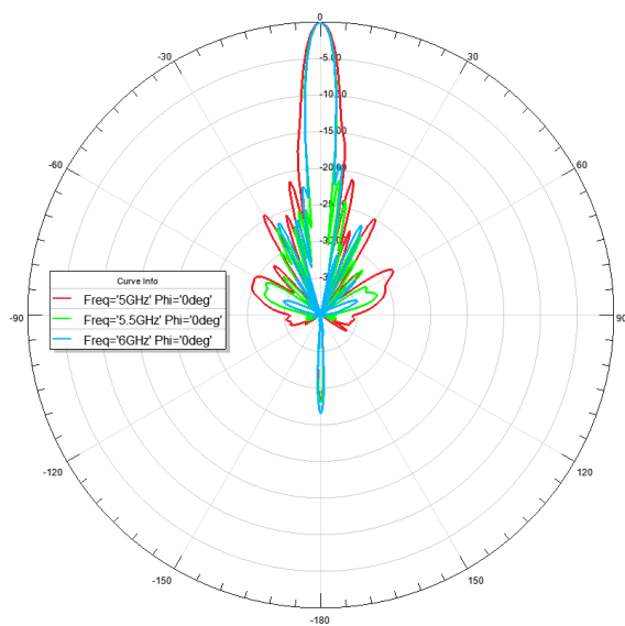
E-plane H-pol
