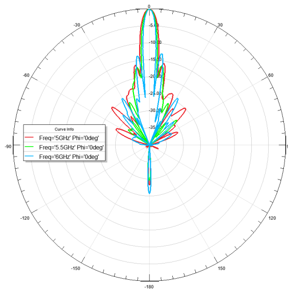
E-plane V-pol
