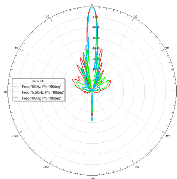
H-plane V-pol
