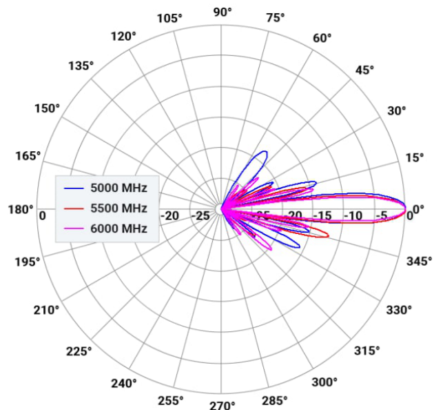
H-plane V-pol
