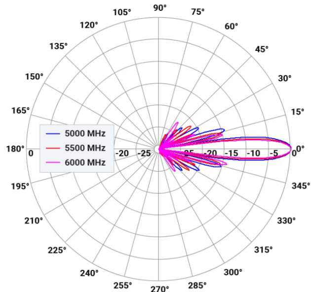
H-plane V-pol
