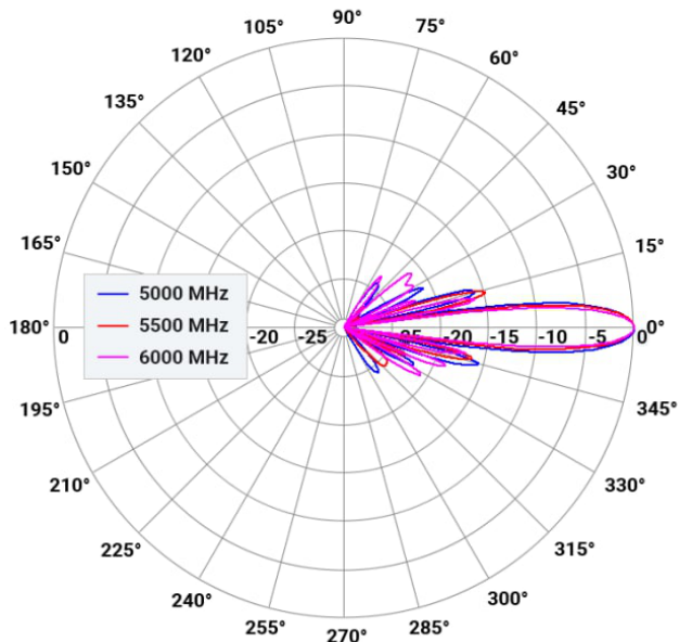
H-plane H-pol
