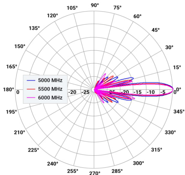
H-plane V-pol
