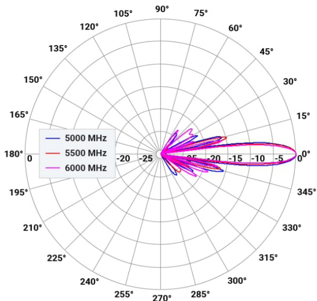
H-plane H-pol
